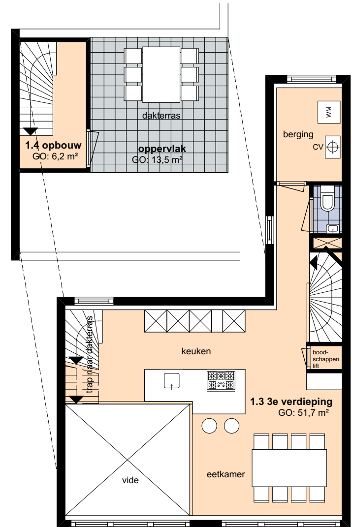
3e verdieping
