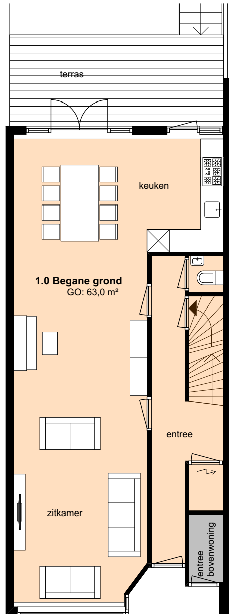
begane grond
