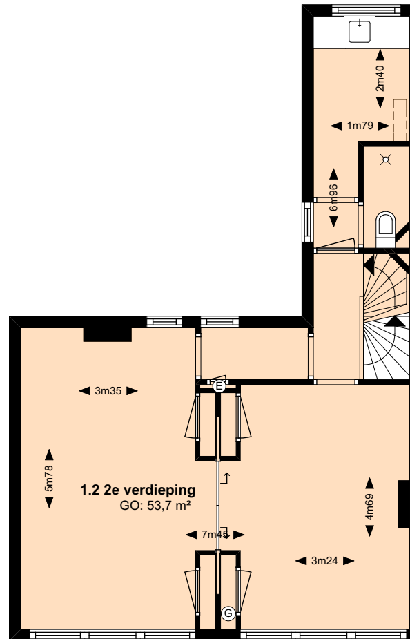
2e verdieping
