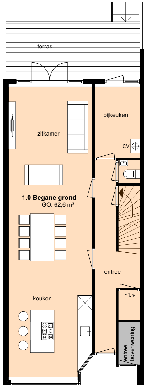
begane grond
