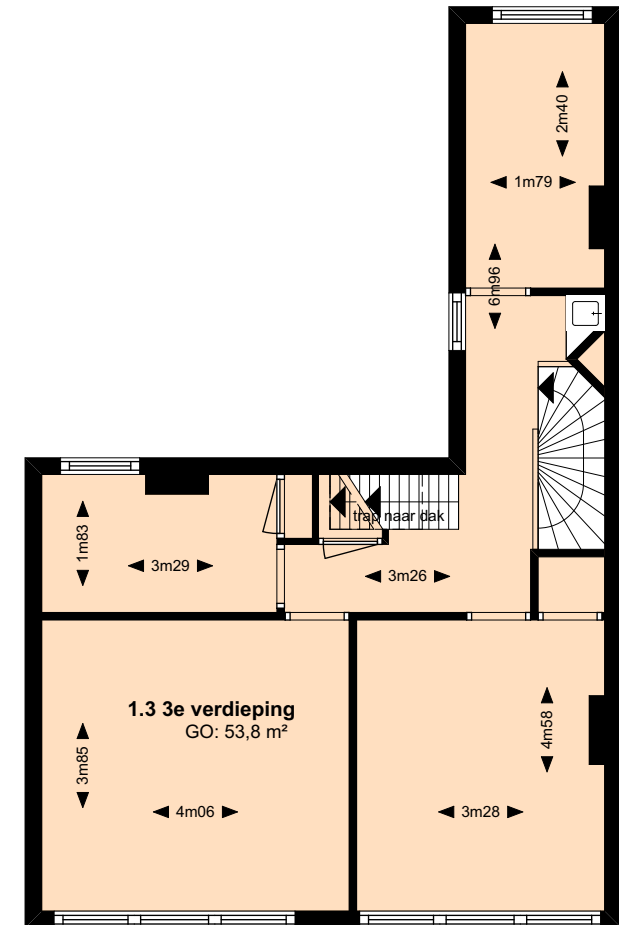
3e verdieping
